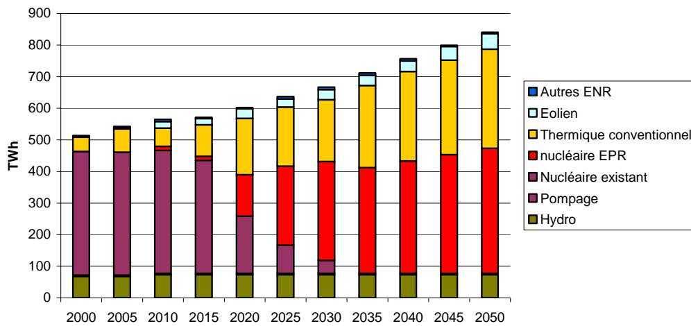
Fig. 13. Mix pour la production d'électricité : politique nucléaire modérée
