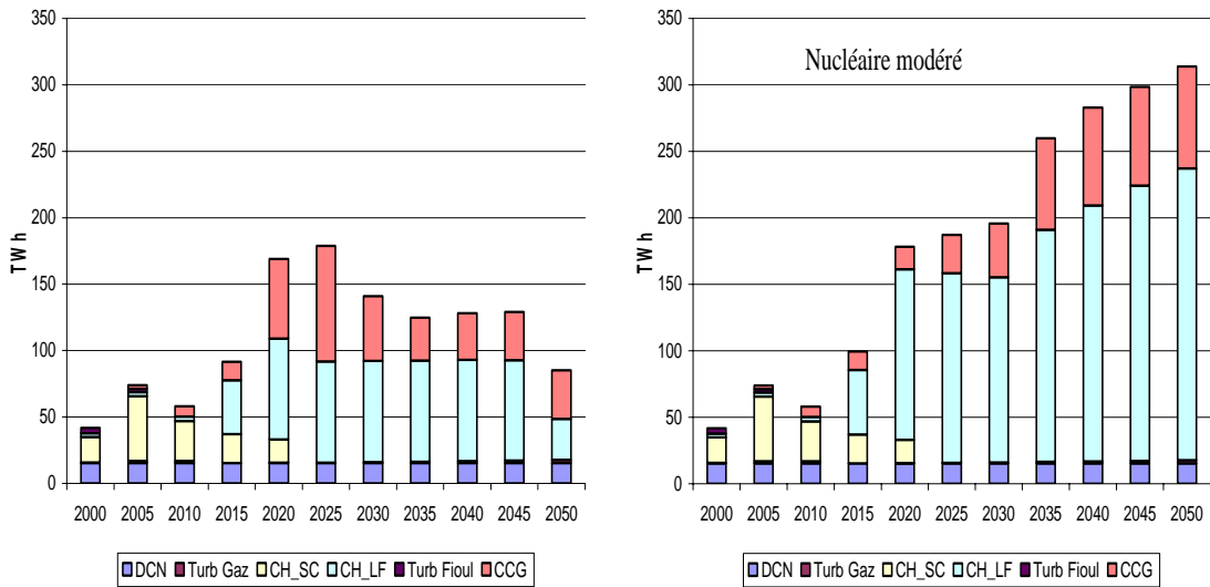
Fig. 14. Mix pour la production thermique avec ou sans contrainte EPR
