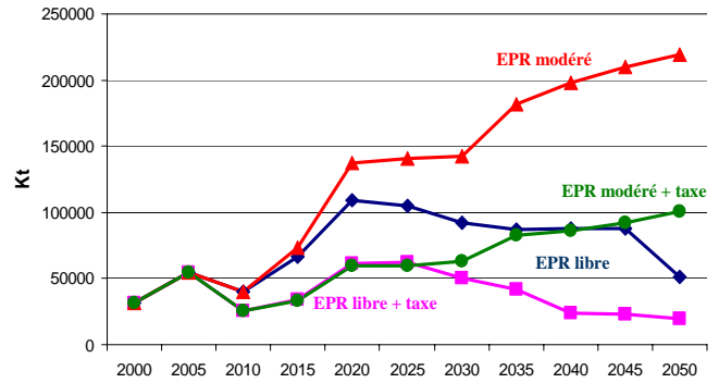
Fig. 12. Effet d’une taxe sur les émissions de CO 2 du secteur de la production d’électricité
