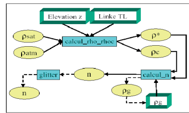
Flowchart of unit «cloud_index»
