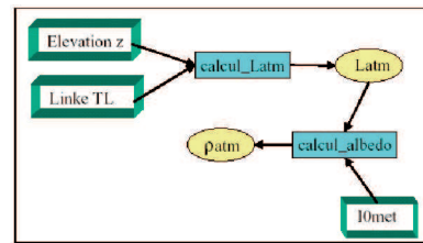
Flowchart of unit «atmosphere»
