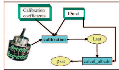
Flowchart of unit «reflectance»
