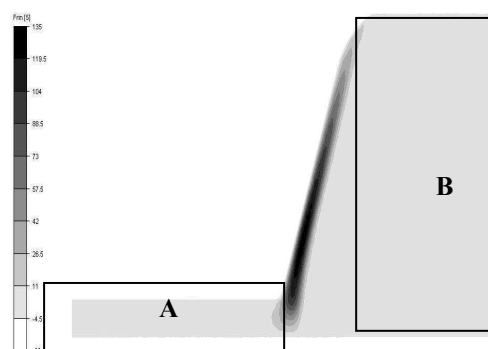
FIG. 7 – vitesse dans le sens transverse de l'écoulement
