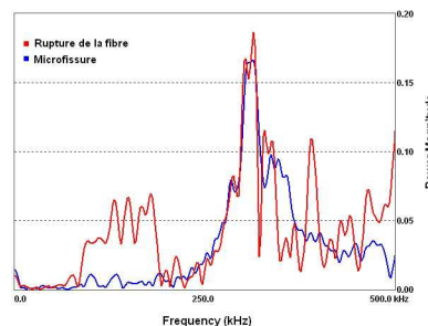
FIG. 1 – Détection par émission acoustique : comparaison des spectres fréquentiels des formes d'ondes des ruptures des fibres et des microfissures.
