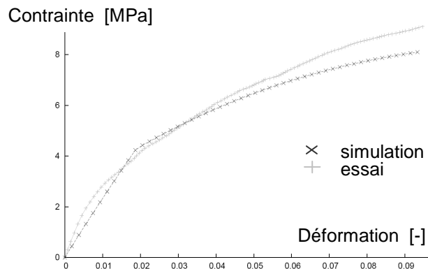
Figure 9. Optimisation des paramètres de plasticité sur l'écouissage à 5.10^{-2} s ^{-1}
