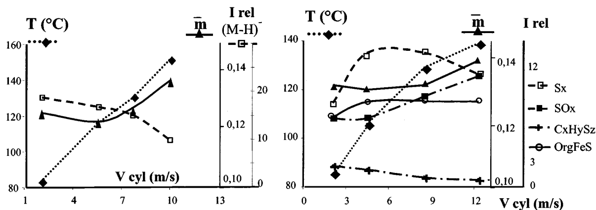
Figure 6. – Laminage de l'acier. Evolution du coefficient de frottement ( \bar{m} ), de la température des bandes (T) et de l'intensité des ions émis par les additifs ( I_{rel} ) en fonction de la vitesse de laminage. Lubrifiant : huile de base additivée de 1 % d'acide stéarique (à gauche) et de 3 % de DTDP (à droite).
