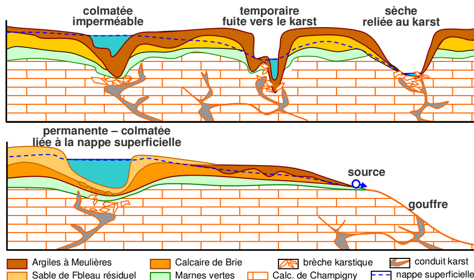
Schéma des configurations hydrologiques et karstiques rencontrées dans le Bois de Barbeau et mises à profit pour le drainage de la forêt.
