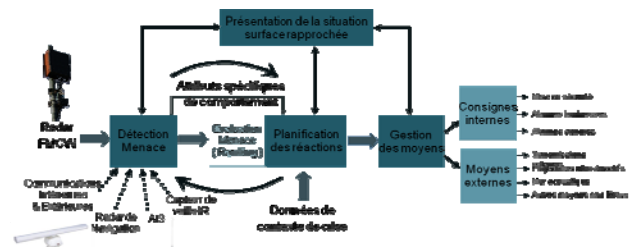
Figure 1 : Schéma fonctionnel
