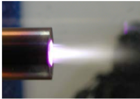
FIG.2. Exemple de post-décharge et son oscillogramme associé. Conditions opératoires : L = 150 \text{ mm} , Q_{\text{air}} = 2 \text{ Nm}^3/\text{h} , P_{\text{elec}} = 1700 \text{ W} .
