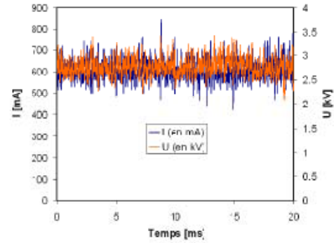
FIG.2. Exemple de post-décharge et son oscillogramme associé. Conditions opératoires : L = 150 \text{ mm} , Q_{\text{air}} = 2 \text{ Nm}^3/\text{h} , P_{\text{elec}} = 1700 \text{ W} .
