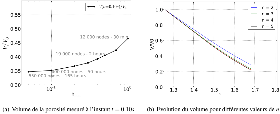
Fig. 4 – Etude de convergence au maillage
