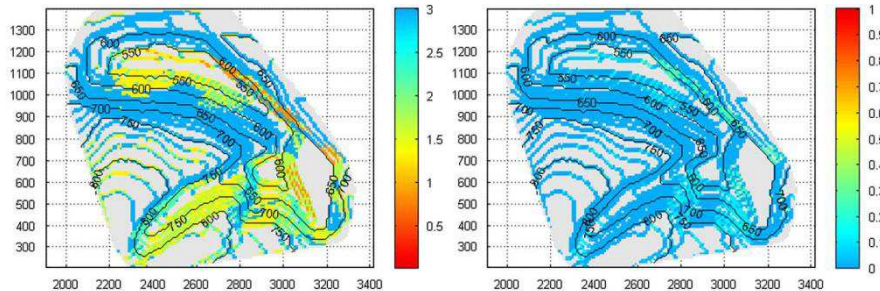
Figure 8 : Analyse de la stabilité structurale des gradins sur la base du MNT de la fosse ultime; carte de facteurs de sécurité (à gauche) et des probabilités de rupture (à droite) [GRE 10].
