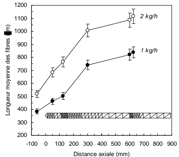
Figure 6. Influence du débit sur l'évolution des longueurs moyennes des fibres à 200 tr/min (introduction avant fusion).
